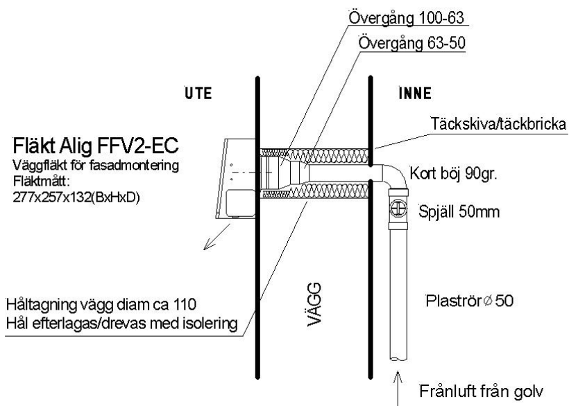
Detalj, FLÄKTMONTAGE ej skala
