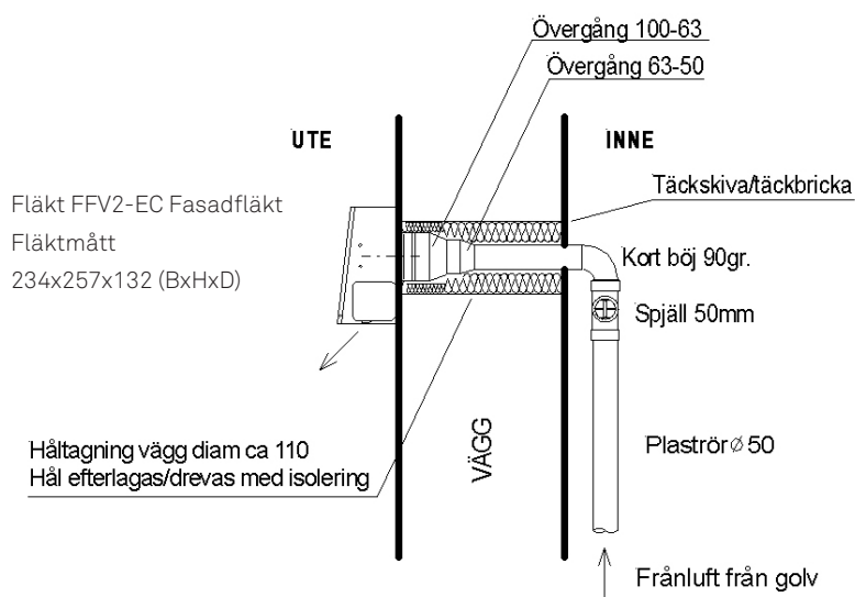
Detalj, FLÄKTMONTAGE ej skala
